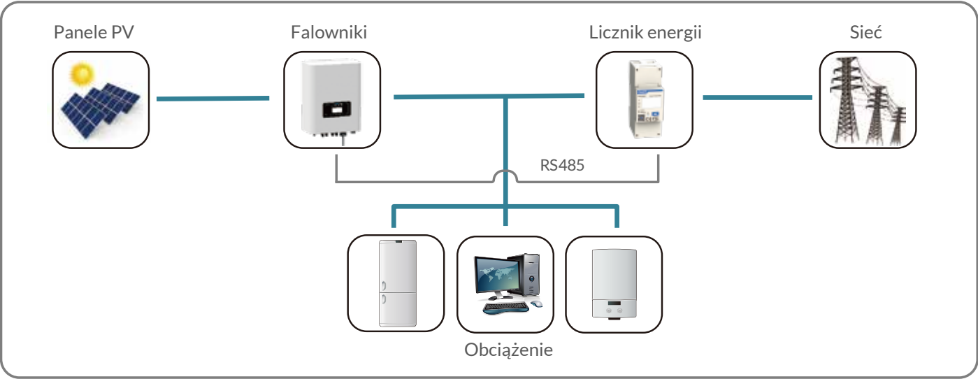
Schemat podłączenia
